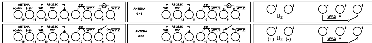
Przykładowe opisy na górnych listwach zaciskowych
